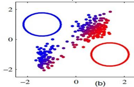
E Step
